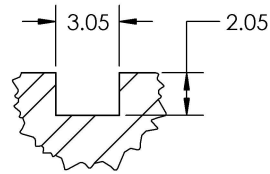
DETALLE B ESCALA 4 : 1
